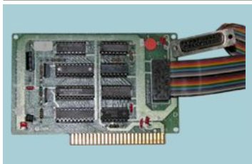
apple II Unidisk/Duodisk 5.25 controller
