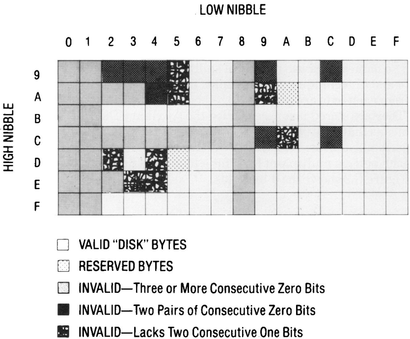
Figure C.4 Valid "Disk Bytes"
