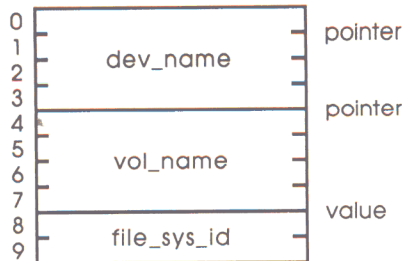
FORMAT ($24) Parameter block
