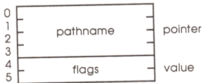
QUIT ($29) Parameter block
