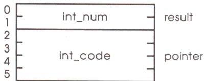
ALLOC_INTERRUPT ($31) Parameter block
