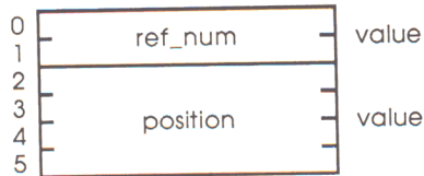
GET_MARK ($17) Parameter block
