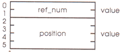
SET_MARK ($16) Parameter block
